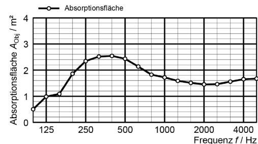
Prüfanordnung 1 artsorber® Deckenabsorber 58, Fläche 2,16 m 2 , Aufbau ohne Wandabstand
