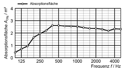
Prüfanordnung 2 artsorber® colour 58, Fläche 2,16 m², Aufbau ohne Wandabstand
