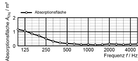
Prüfanordnung 1 artbass whiteboard 58, Whiteboard magnetisch Fläche 1,51 m², Aufbau ohne Wandabstand
