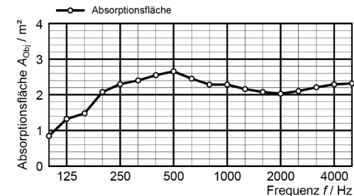
Prüfanordnung 2 artsorber® print 89, Fläche 2,13 m 2 , Aufbau ohne Wandabstand
