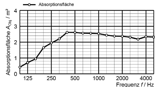
Prüfanordnung 1 artsorber® print 58, Fläche 2,16 m 2 , Aufbau ohne Wandabstand
