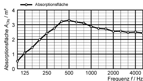
Prüfanordnung 1 Deckensegel metal 50, Fläche 2,16 m², Aufbau mit 100mm Abstand
