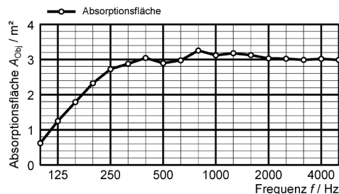
Prüfanordnung 2 Deckensegel metal 50, Fläche 2,16 m², Aufbau mit 300mm Abstand
